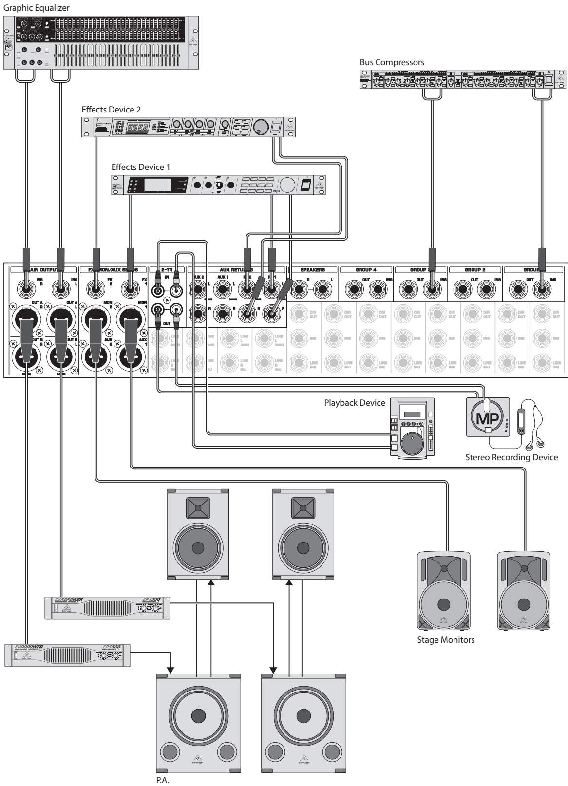
Afb. 2.2: Bekabeling van de kanalen (uitgangen)
