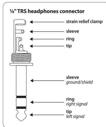
Afb. 3.5: Koptelefoon-stereoklinkerstekker
