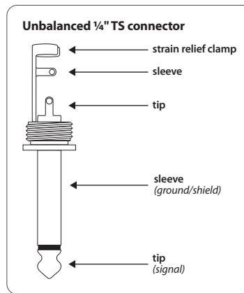
Afb. 3.3: 6,3 mm monoklinkerstekker
