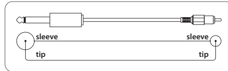
Kuva. 4.4: Sovitinkaapeli, mono
