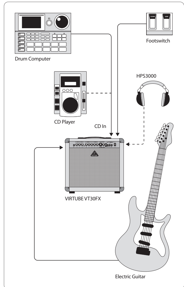
Kuva. 3.1: VIRTUBE-vakiokokoonpano
