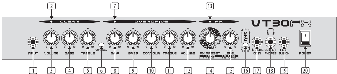
Kuva. 2.1: VIRTUBE-vahvistimen käyttöelementit (etupuoli)
