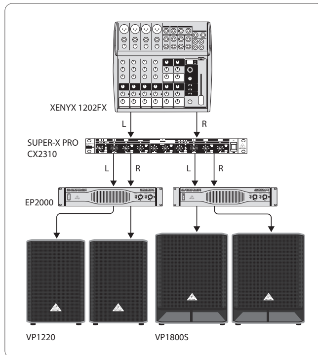
図 5.3: フルレンジ・ステレオ・オペレーションとサブウーファー
