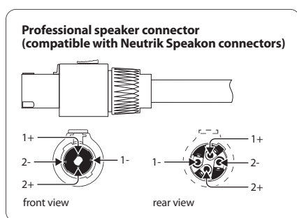
図. 2.2: プロフェッショナル・ラウドスピーカー・コネクタ
