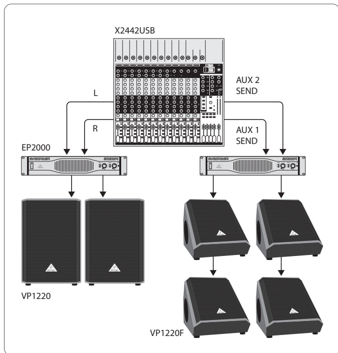
図 5.2: フルレンジ・ステレオ・オペレーションとフロアモニター
