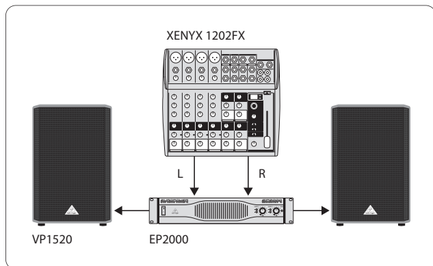
図 5.1: フルレンジ・ステレオ・オペレーション
