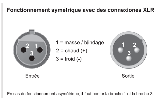
Fig. 5.2 : Connecteur XLR
