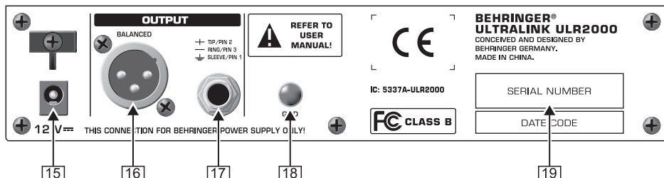
Fig. 2.3 : Panneau arrière de l'ULR2000
