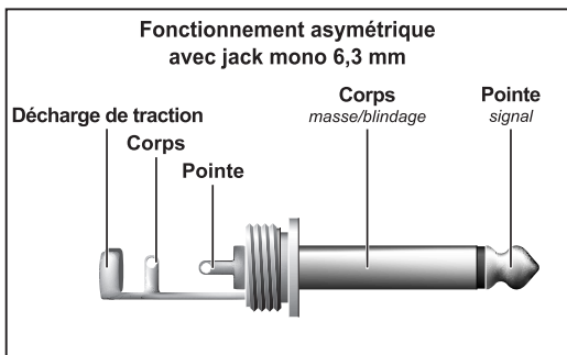
Fig. 5.3 : Jack mono de 6,3 mm
