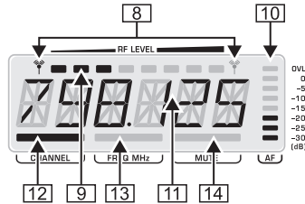
Fig. 2.2 : Détail de l'afficheur de l'ULR2000
