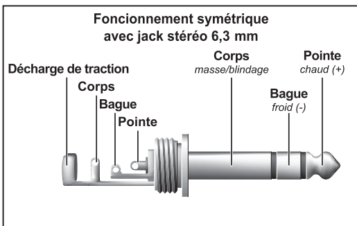
Fig. 5.4 : Jack stéréo de 6,3 mm
