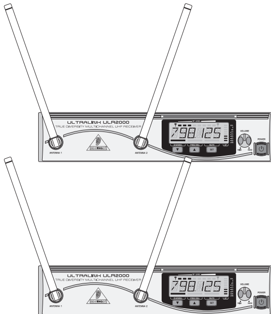
Fig. 5.1 : Disposition des ULR2000 montés les uns au-dessus des autres
