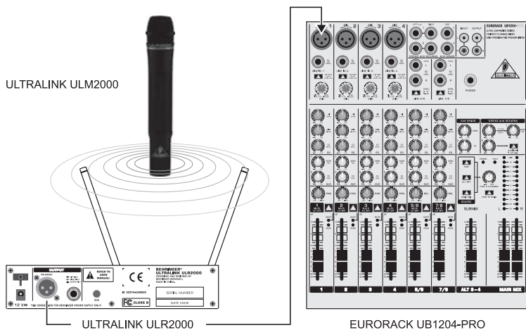
Fig. 4.1 : Câblage du récepteur ULR2000 et du micro ULM2000
