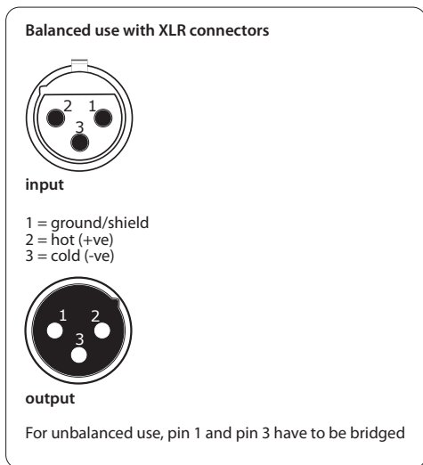
Fig. 5.1: XLR-verbindingen
