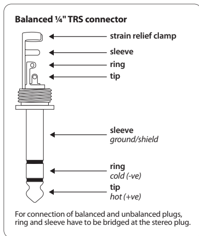
図 4.2: ステレオジャックプラグ付き左右対称ジャックケーブル
