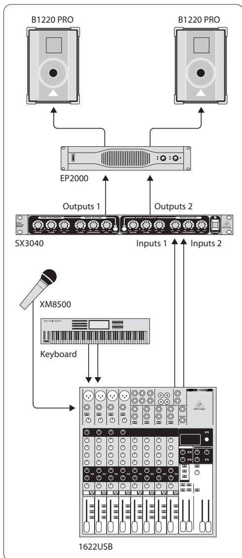
図 3.1: SX3040 を音響装置と併用する場合
