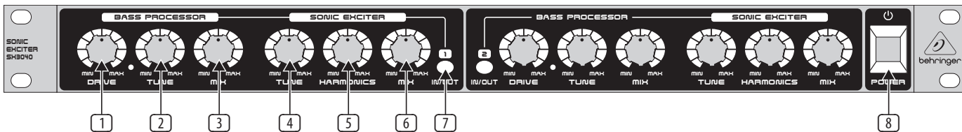
図 2.1: 前面の操作エレメント
