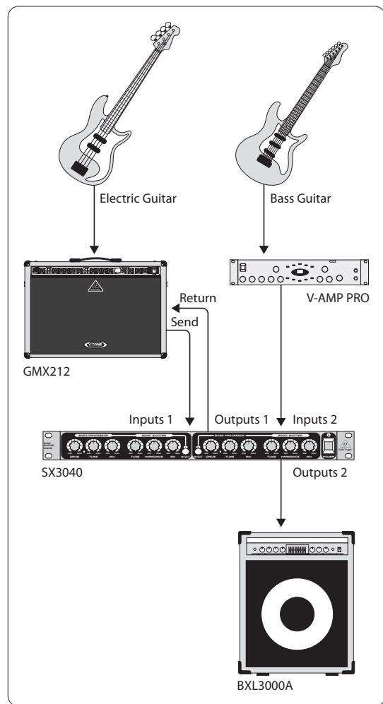
図 3.3: ギターアンプと併用した場合の SX3040
