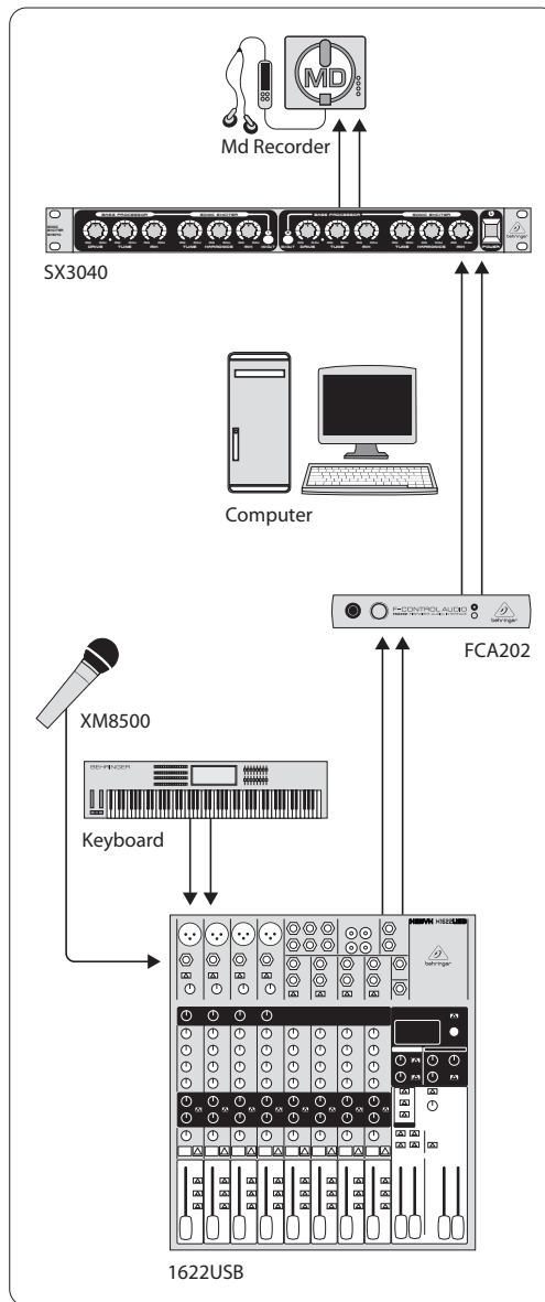
図 3.2: SX3040 のスタジオでの使用
