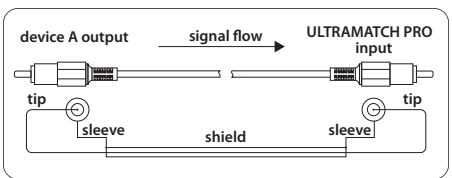
Fig. 4.4: Modo de ligação assimétrica do ULTRAMATCH PRO
