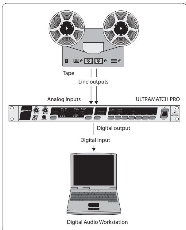
Fig. 3.2: Exemplo de conversão A/D de gravações em fitas magnéticas antigas
