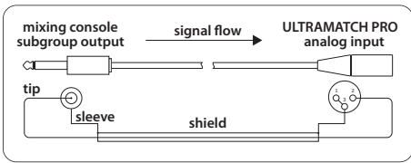
Fig. 4.1: Transmitir de forma assimétrica para o ULTRAMATCH PRO
