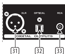
Fig. 2.8: Saídas digitais do ULTRAMATCH PRO
