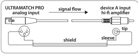
Fig. 4.2: Receber de forma assimétrica do ULTRAMATCH PRO
