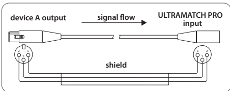
Fig. 4.3: Modo de ligação simétrica do ULTRAMATCH PRO
