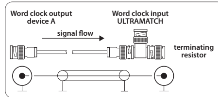
Fig. 4.6: Modo de ligação assimétrico (terminação) da entrada do Wordclock no ULTRAMATCH PRO
