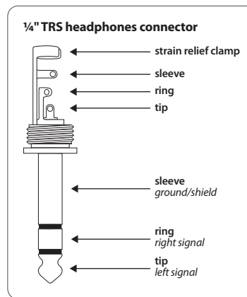
Fig. 4.7: Ocupação correcta para a alimentação para os auscultadores
