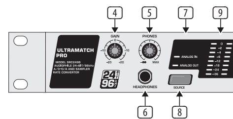
Fig. 2.2: Elementos de comando da secção de entrada
