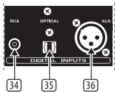
Fig. 2.9: Entradas digitais
