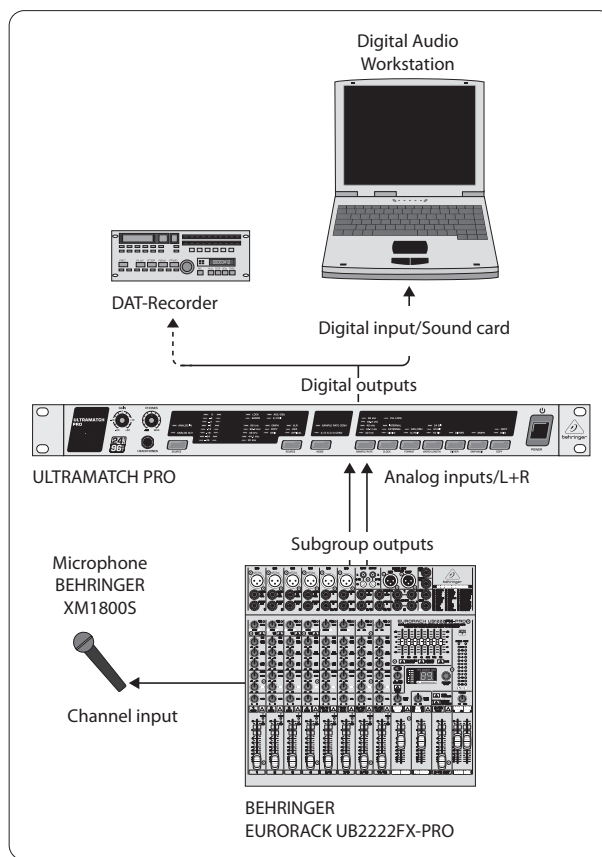
Fig. 3.1: Exemplo conversão A/D de um sinal de microfone
