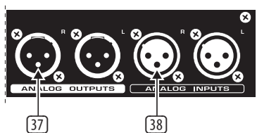
Fig. 2.10: Saídas/entradas analógicas
