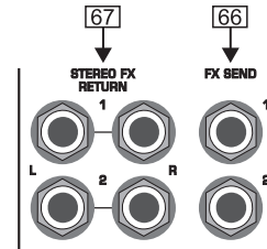
Kuva 2.26: FX Send- ja Return-liitännät
