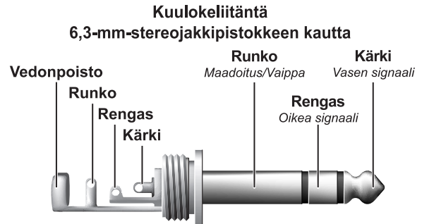
Kuva 5.6: Kuuloke-stereojakkipistoke
