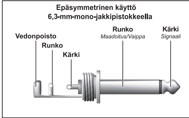
Kuva 5.1: 6,3 mm monojakkipistoke
