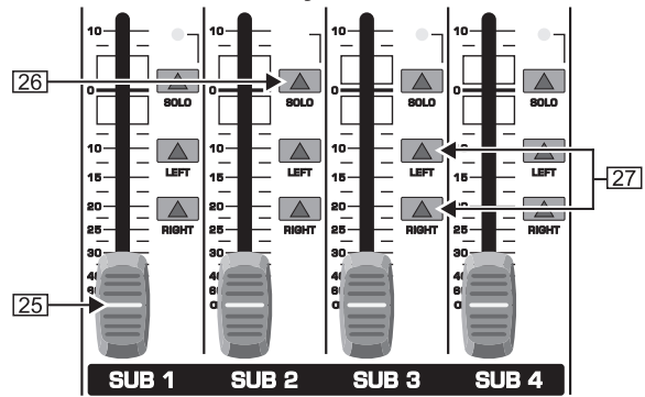
Kuva 2.9: Alaryhmät 1 - 4
