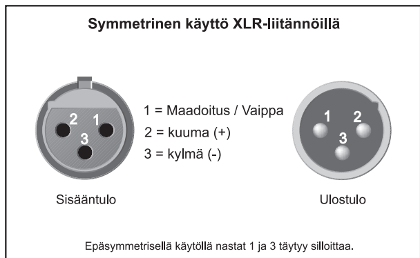
Kuva 5.4: XLR-liitännät
