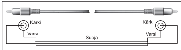
Kuva 5.3: Cinch-kaapeli
