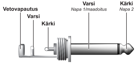
Kuva 5.5: Monojakkiliitin jalkapainikkeelle
