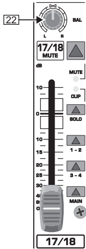
Kuva 2.7: Kanavan faderi, balanssisäädin, vaimennuskytkin jne.
