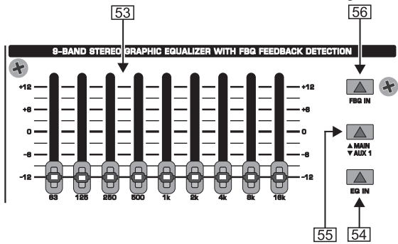
Kuva 2.24: Graafinen stereokorjain
