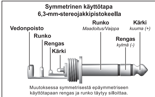
Kuva 5.2: 6,3 mm stereojakkipistoke
