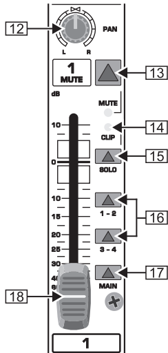
Kuva 2.4: Kanavafaderi, yleissäädin, vaimennuskytkin jne.
