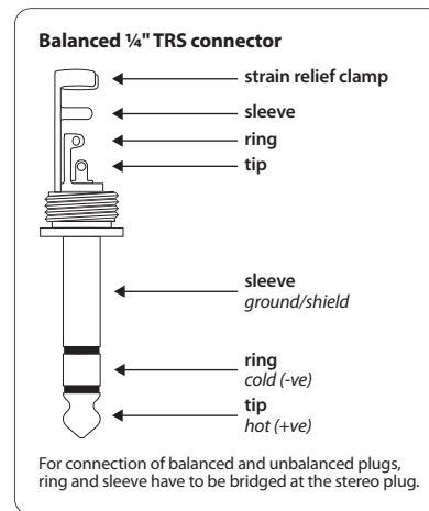
Afb. 5.1: 6,3-mm-stereoklinkerstekker
