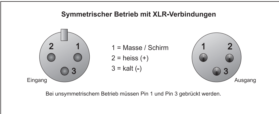
Abb. 8.1: Verschiedenen Steckertypen
