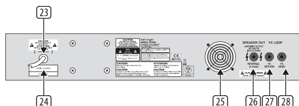
Fig. 2.2: Eléments de contrôle du GUITAR COMBO (panneau arrière)
