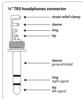
Fig. 4.2: Jack stéréo de 6,3 mm
