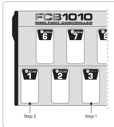
Afb. 2.2: Bedieningsstappen ter selectie van een preset bij ingeschakelde DIRECT SELECT
