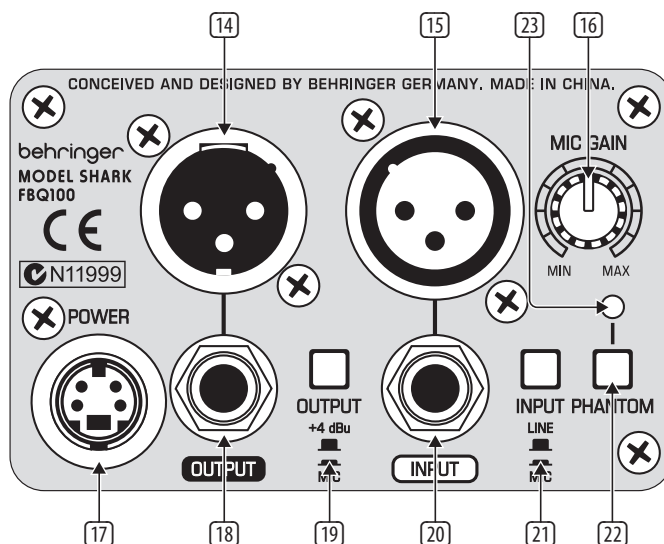
Fig. 1.2: Los elementos de mando y conexiones en el lado posterior del FBQ100
