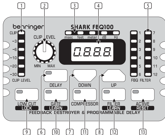
Fig. 1.1: Los elementos de mando del lado frontal del DSP 110.
