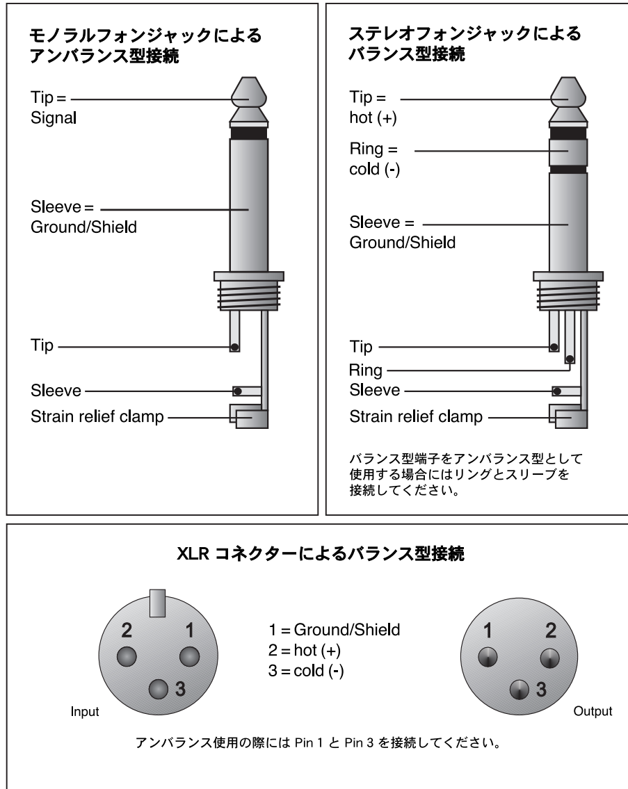
図 3.5: 各種プラグの比較
