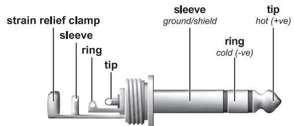
図 4.5: 6.3-mm ステレオ・フォンジャック
