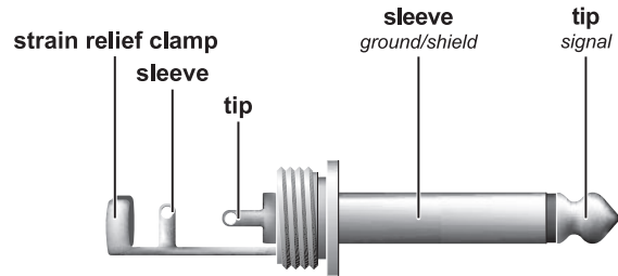
図 4.4: 6.3-mm モノ・フォンジャック
