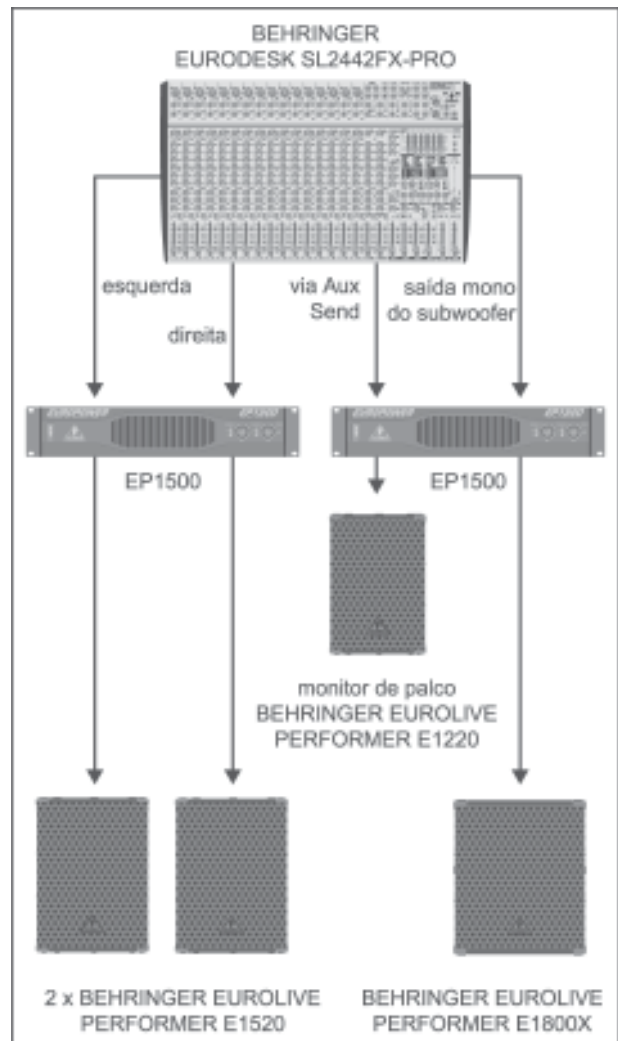
Fig. 6.1: Funcionamento em estéreo com monitor de palco e subwoofer
