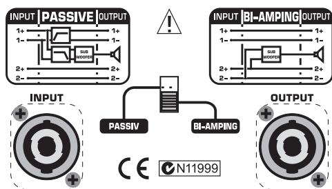
Fig. 1.1: Área de ligação do subwoofer (E1800X)
