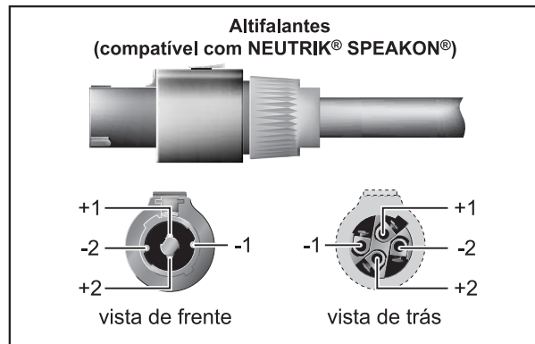
Fig. 1.2: Ficha Speakon®
