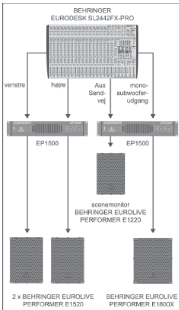
Fig. 6.1: Stereodrift med scenemonitor og subwoofer
