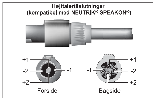
Fig. 1.2: Speakon®-stik
