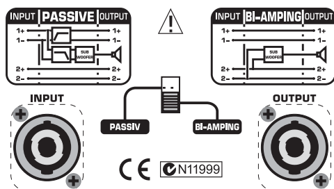
Fig. 1.1: Tilslutning af Subwoferen (E1800X)
