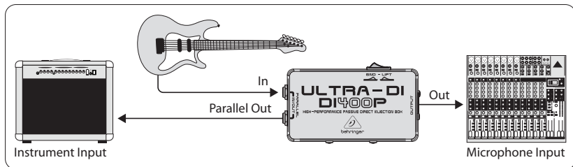
Bild 2: Gitarr → DI-box → gitarrförstärkare/mixerbord
