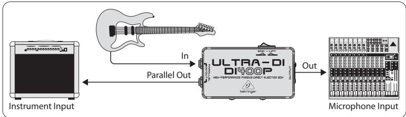
Kuva 2: Kitara → DI-boksi → Kitaravahvistin/Mikseripöytä
