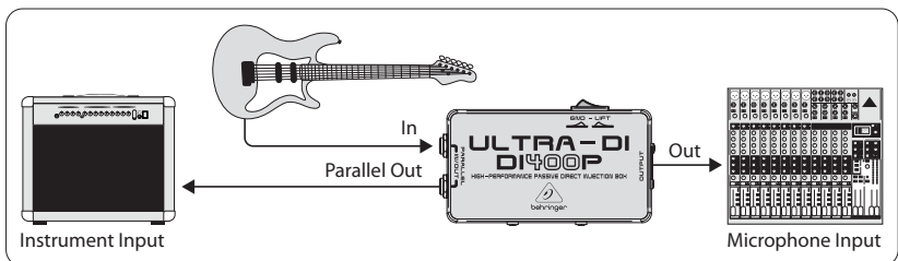
Afb. 2: Gitaar → DI-box → gitaarversterker/mengpaneel
