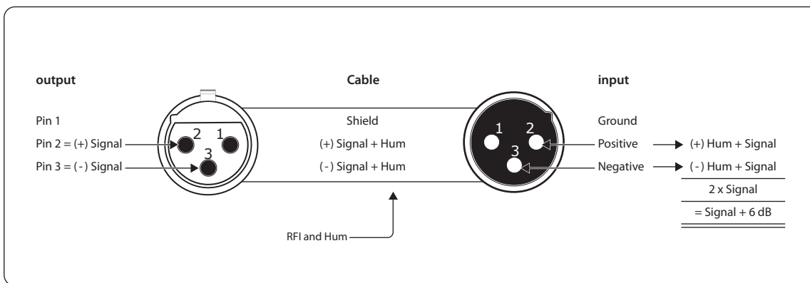
Abb. 4.1: Kompensation von Störungen bei symmetrischem Betrieb
