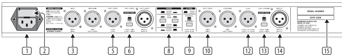
Abb. 2.4: Aktive Bedienelemente auf der Rückseite der SUPER-X PRO in der Stereo 2-Weg Betriebsweise
