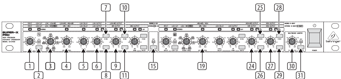
Abb. 2.9: Aktive Bedienelemente auf der Frontseite der SUPER-X PRO in der Mono 4-Weg Betriebsweise
