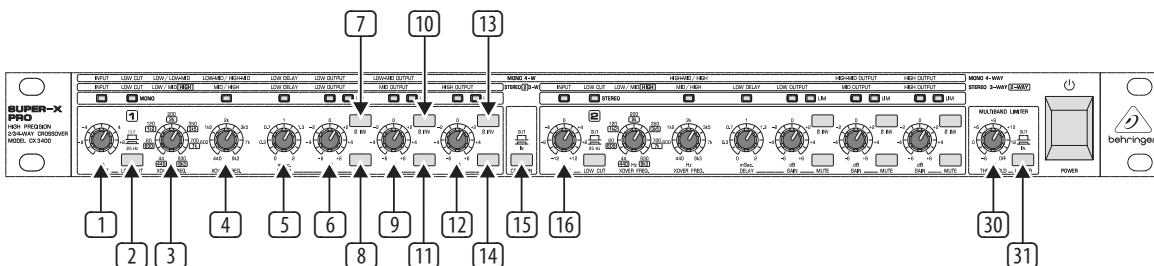
Abb. 2.6: Aktive Bedienelemente auf der Frontseite der SUPER-X PRO in der Stereo 3-Weg Betriebsweise
