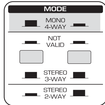
Abb. 2.8: Richtige Anwahl der beiden MODE -Schalter für die Mono 4-Weg Betriebsweise
