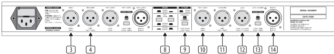
Abb. 2.7: Aktive Bedienelemente auf der Rückseite der SUPER-X PRO in der Stereo 3-Weg Betriebsweise
