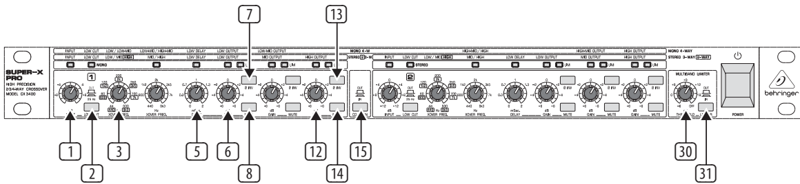
Abb. 2.3: Aktive Bedienelemente auf der Frontseite der SUPER-X PRO in der Stereo 2-Weg Betriebsweise
