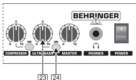
Fig. 2.7: Funzione ULTRABASS (non BXL450 e BXL450A)
