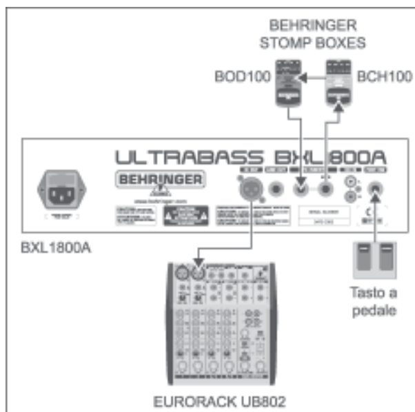
Fig. 4.2: Setup avanzato (qui BXL1800A)
