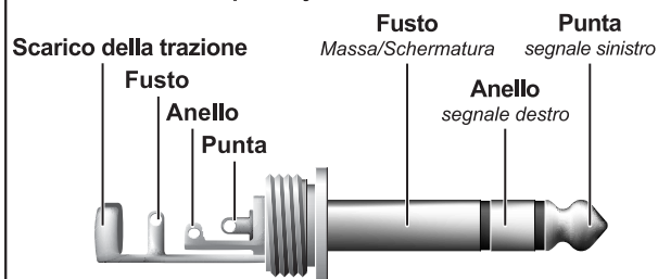
Fig. 5.3: Spina jack stereo da 6,3 mm per PHONES
