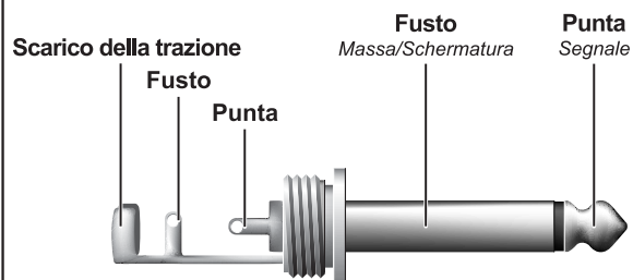
Fig. 5.2: Presa jack mono 6,3 mm
