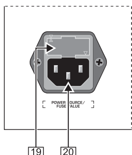
Fig. 2.5: Supporto di sicurezza ed attacco di ingresso IEC (lato posteriore)
