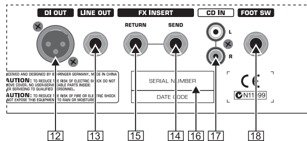
Fig. 2.4: I collegamenti posteriori (BXL1800, BXL3000, BXL1800A e BXL3000A)
