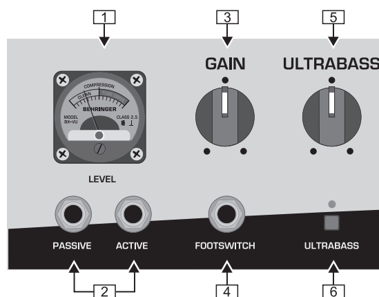
Fig. 2.1: Elementos de comando no lado dianteiro do aparelho (secção 1)
