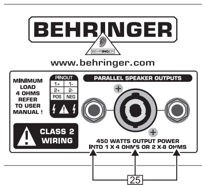
Fig. 2.5: Parte traseira do BX4500H (secção 2)
