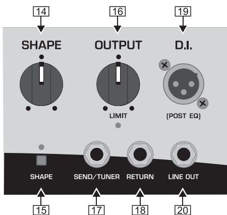
Fig. 2.3: Elementos de comando no lado dianteiro do aparelho (secção 3)
