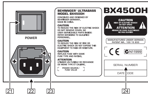
Fig. 2.4: Parte traseira do BX4500H (secção 1)
