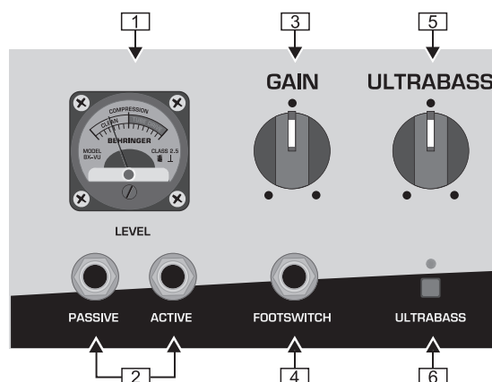
Fig. 2.1: Lato frontale del BX4500H (sezione 1)
