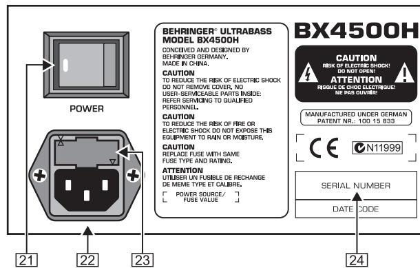
Fig. 2.4: Retro del BX4500H (sezione 1)
