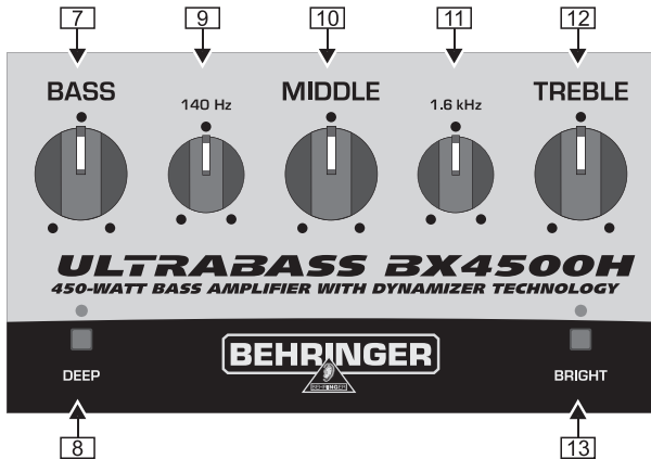
Fig. 2.2: Lato frontale del BX4500H (sezione 2)
