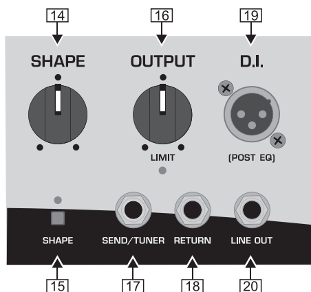
Fig. 2.3: Lato frontale del BX4500H (sezione 3)
