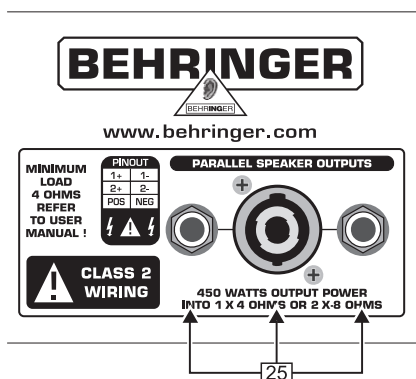
Fig. 2.5: Retro del BX4500H (sezione 2)
