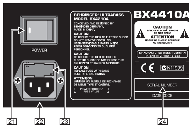
Fig. 2.4: BX4410/BX4410As bagside (udsnit 1)
