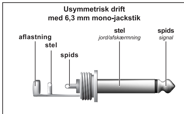
Fig. 7.1: 6,3 mm mono-jackstik
