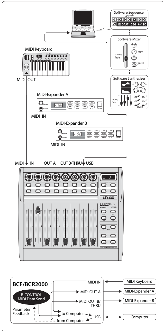
Рис. 4.3: Маршрутизация и использование в режиме USB 3
