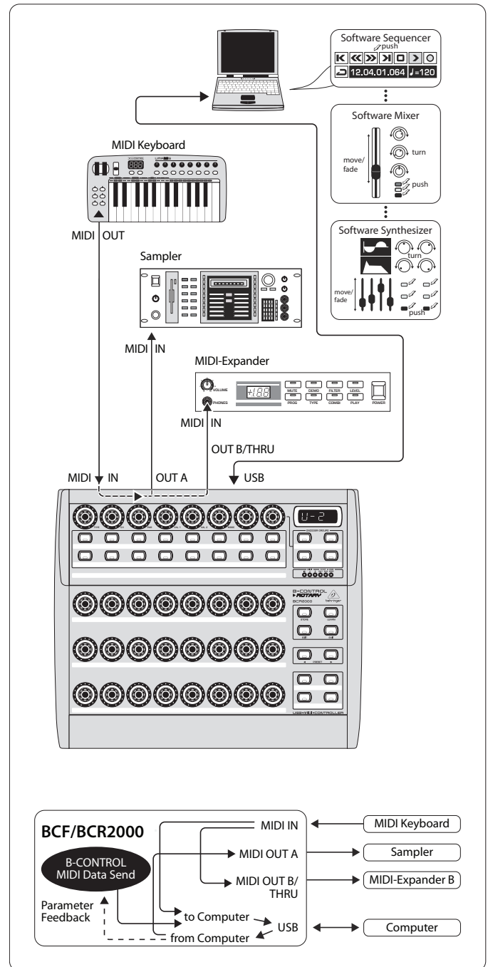
Рис. 4.2: Маршрутизация и использование в режиме USB 2
