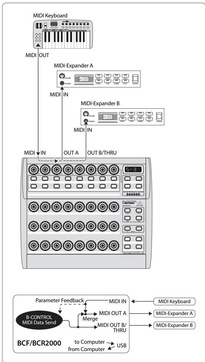
Fig. 4.8 : Utilisation et routing du mode Stand-Alone 3
