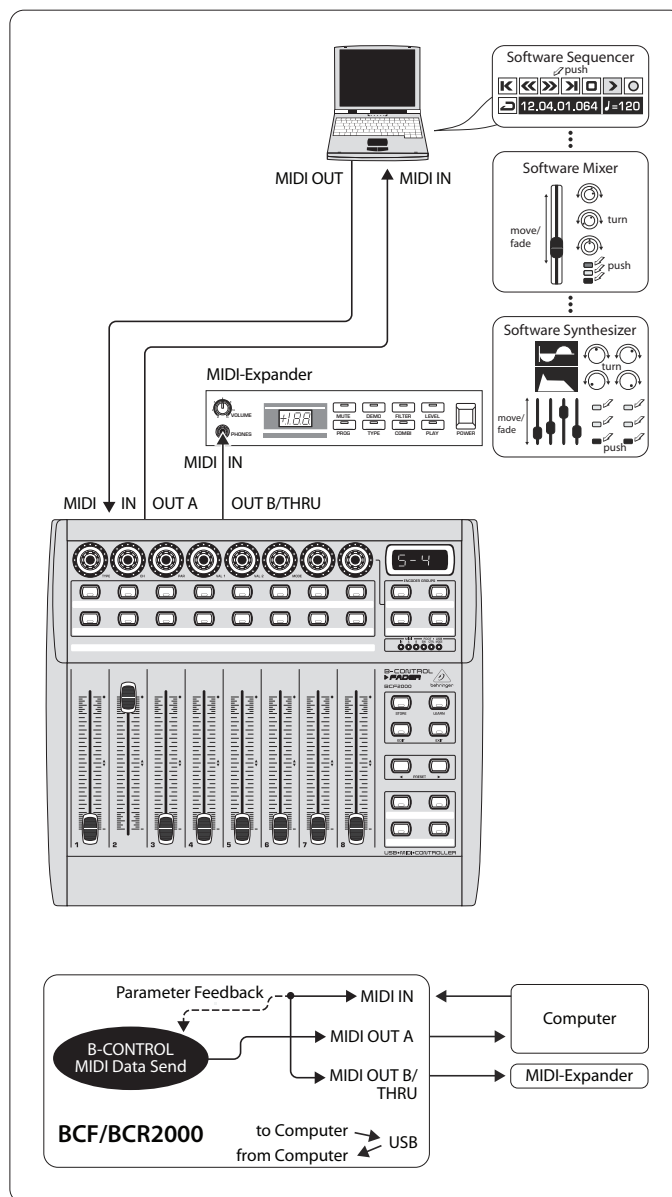
Fig. 4.9 : Utilisation et routing du mode Stand-Alone 4
