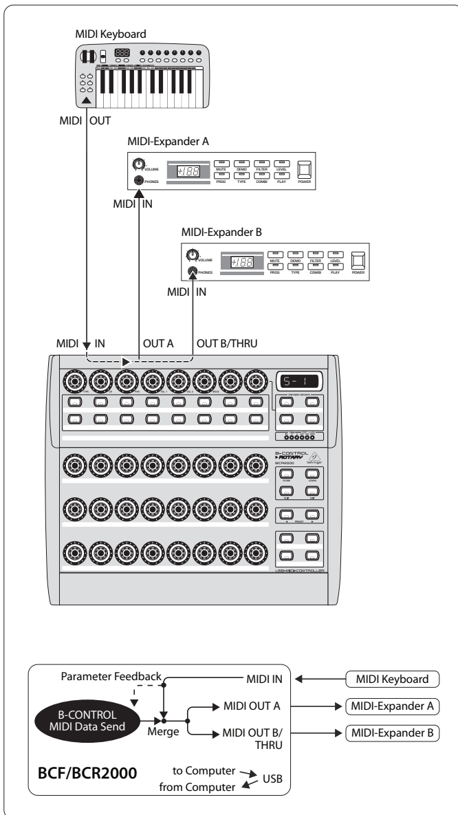
Fig. 4.6 : Routing et utilisation du mode Stand-Alone 1
