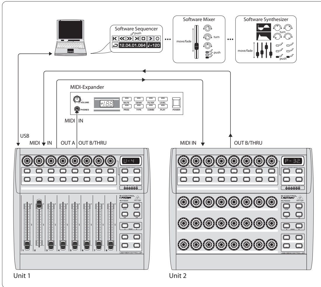
Fig. 4.4 : Utilisation en mode USB 4 (Expanded)
