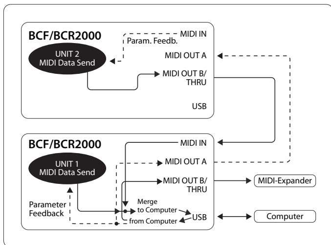
Fig. 4.5 : Routing en mode USB 4
