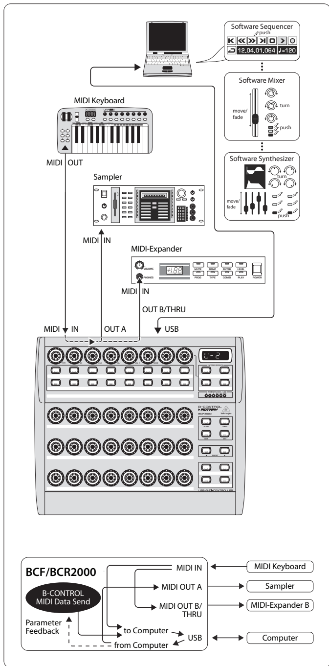
Fig. 4.2 : Routing et utilisation du mode USB 2
