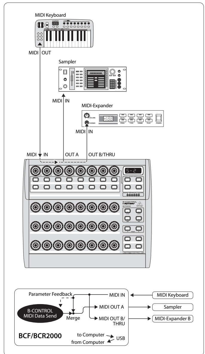
Fig. 4.7 : Routing et utilisation du mode Stand-Alone 2
