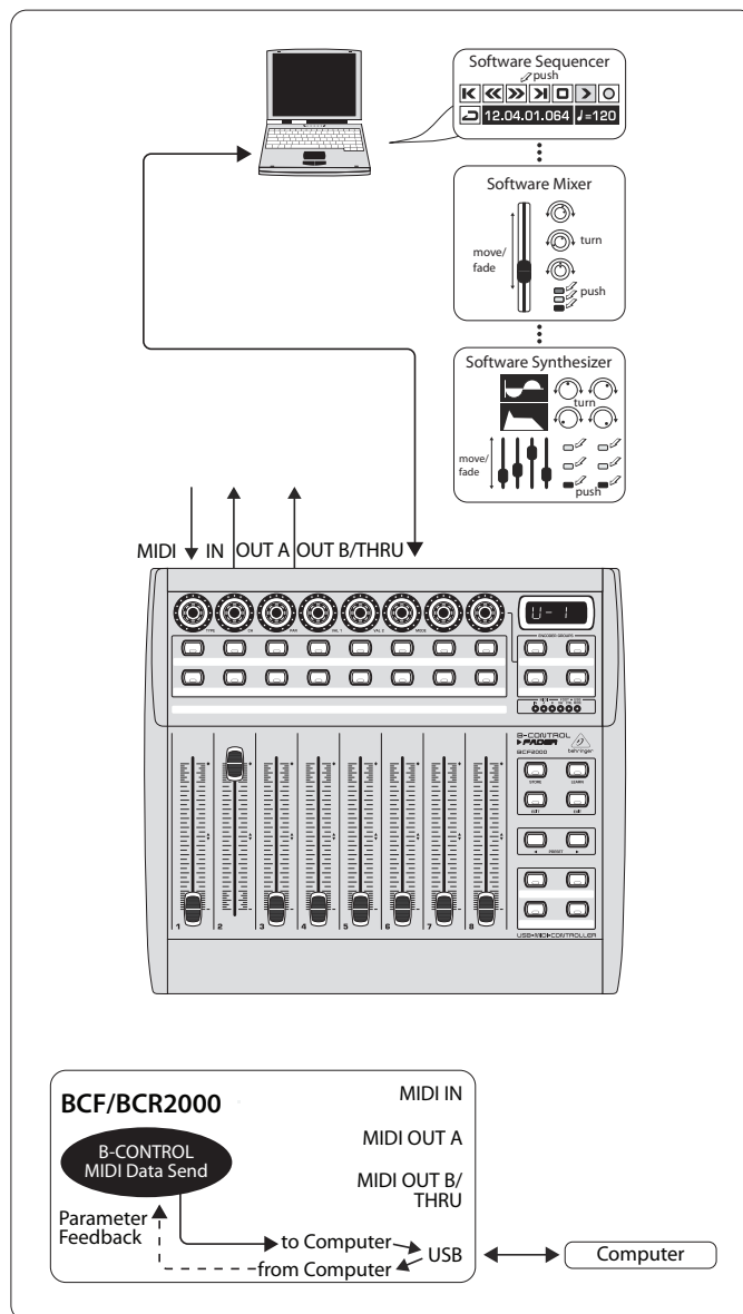
Fig. 4.1 : Routing et utilisation du mode USB 1
