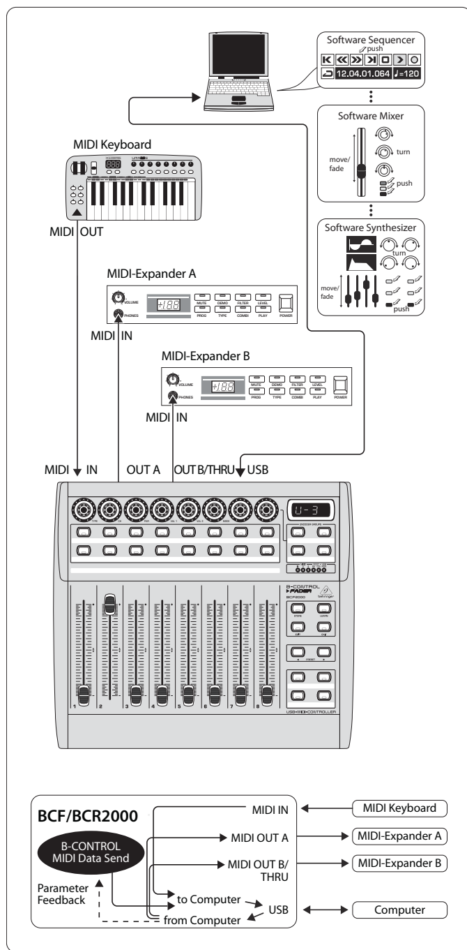
Fig. 4.3 : Routing et utilisation du mode USB 3
