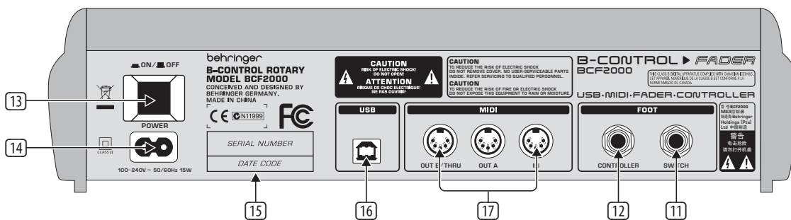
Fig.3.2 : La panneau arrière du BCF2000 (éléments 13 à 17) identiques à ceux du BCR2000)
