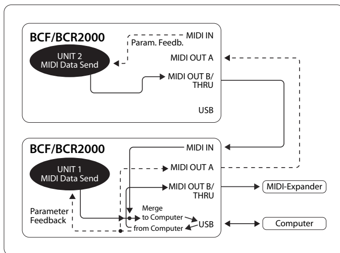
Fig. 4.5: Routing nel modo USB 4
