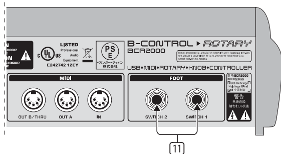
Fig. 3.3. I connettori dei pedali del BCR2000
