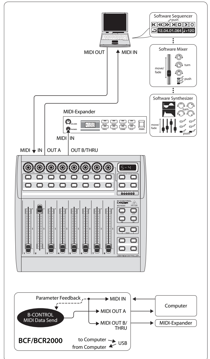
Fig. 4.9: Applicazione e routing nel modo Stand Alone 4
