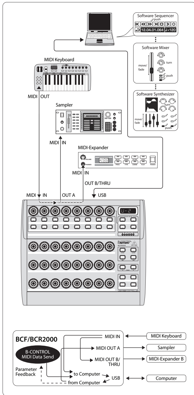
Fig. 4.2: Routing e applicazione nel modo USB 2
