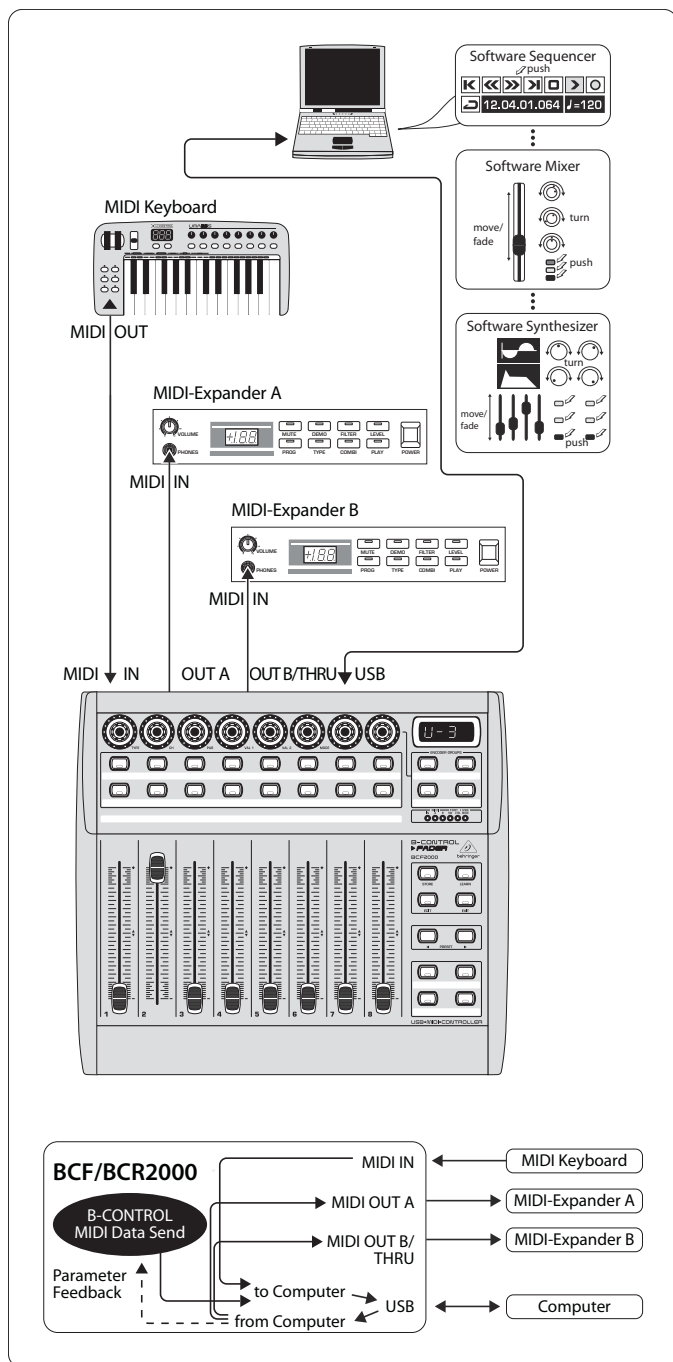
Fig. 4.3: Routing e applicazione nel modo USB 3
