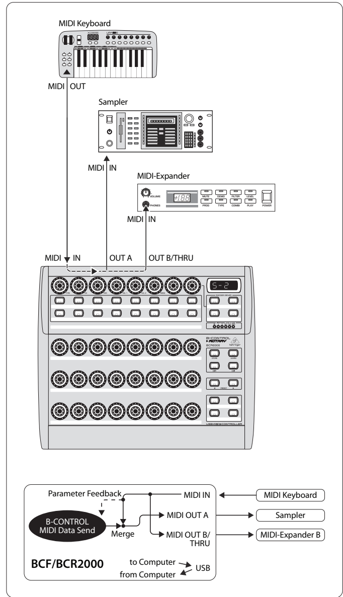
Fig. 4.7: Routing e applicazione nel modo Stand Alone 2
