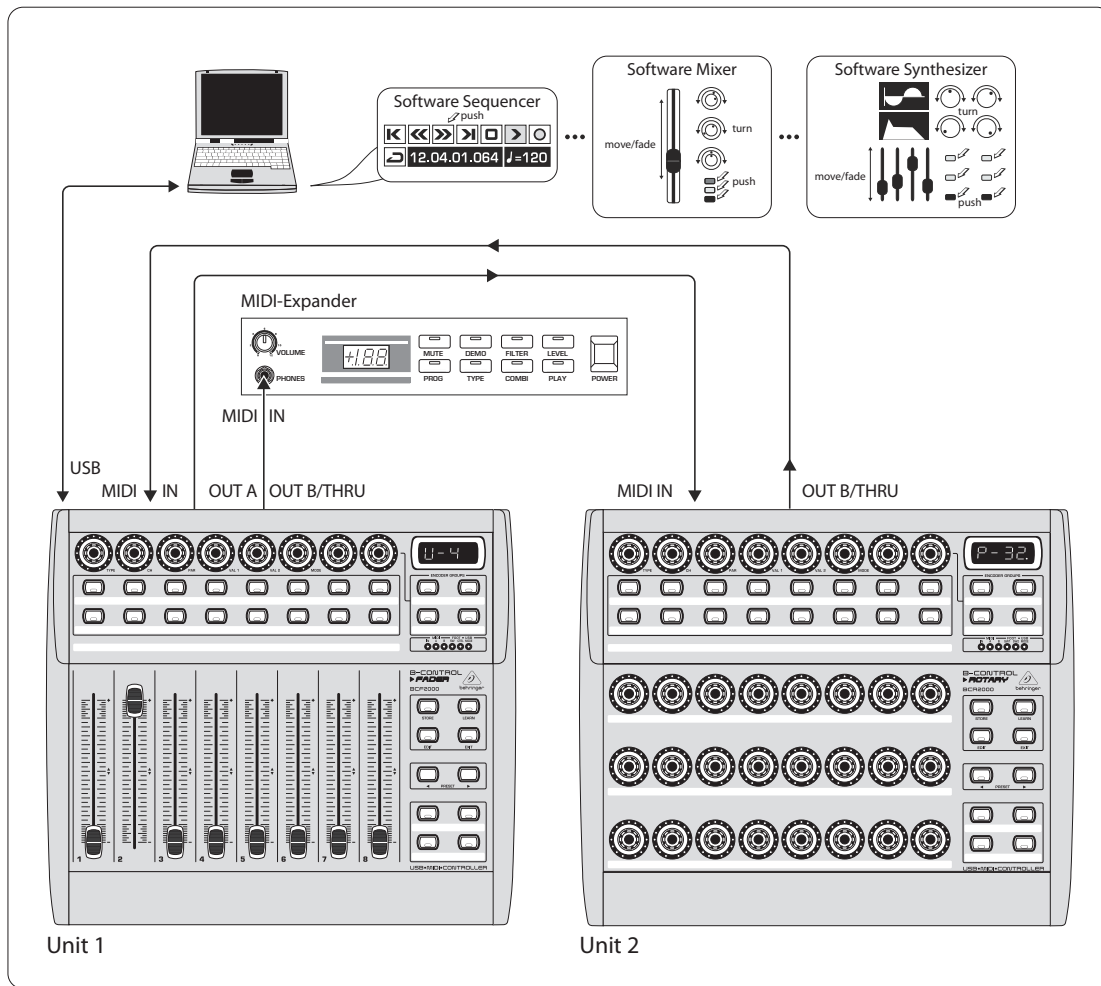
Fig. 4.4: Applicazione nel modo USB 4 (Expanded)
