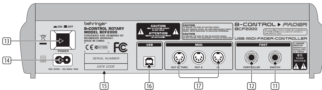
Fig. 3.2. Il retro del BCF2000 (gli elementi di comando da 13 a 17 coincidono con quelli BCR2000)
