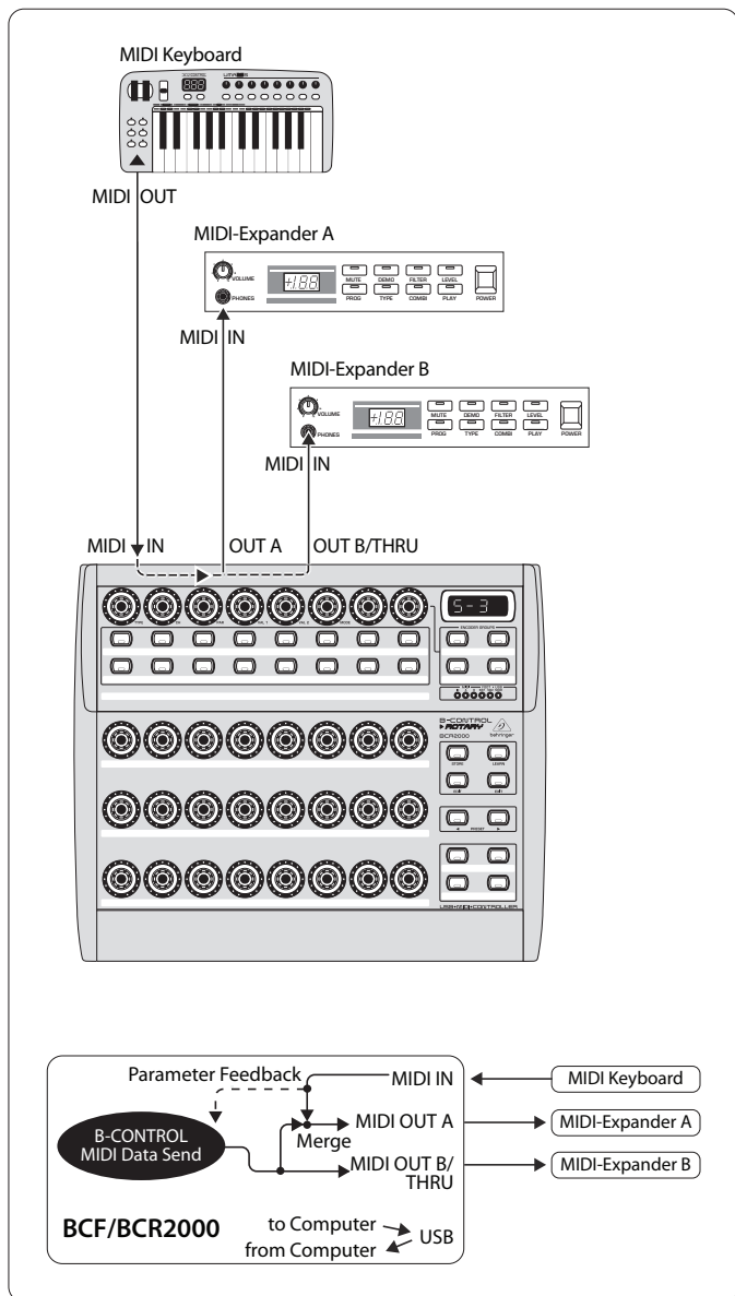
Fig. 4.8: Applicazione e routing nel modo Stand Alone 3
