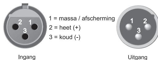
Afb. 4.1: XLR-aansluitingen
