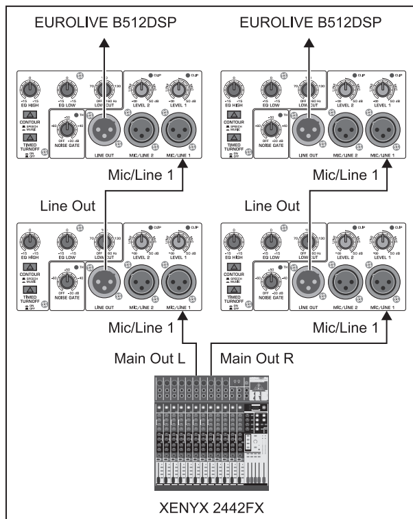
Afb. 3.3: Aaneenschakeling van meerdere B512DSP's
