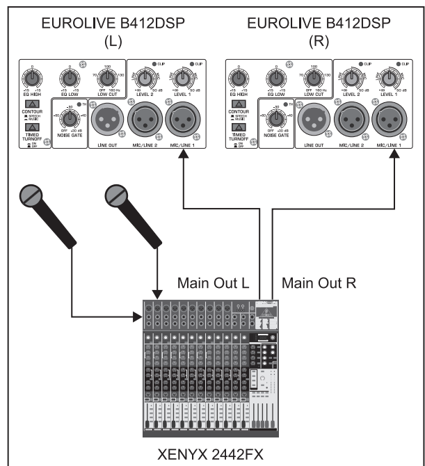
Fig. 3.2 : Câblage d'une table de mixage
