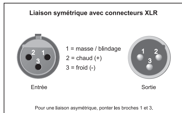
Fig. 4.1: Connecteurs XLR
