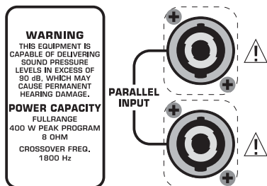
Kuva 1.1: B1520 PRO -kaiuttimen liitäntäalue (sama kuin B1220 PRO -kaiuttimessa)
