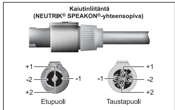
Kuva 1.3: Speakon®-pistoke
