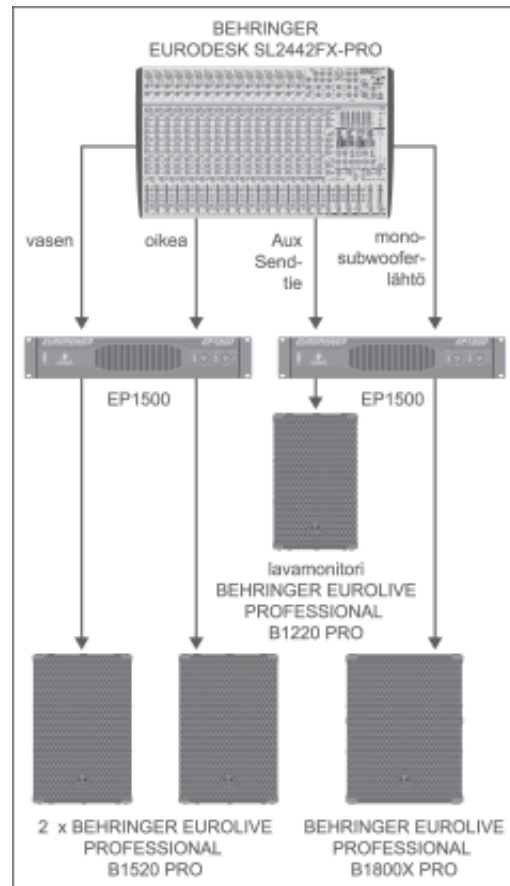
Kuva 6.1: Stereokäyttö: rinnakkainen lavamonitorijärjestelmä ja subwoofer
