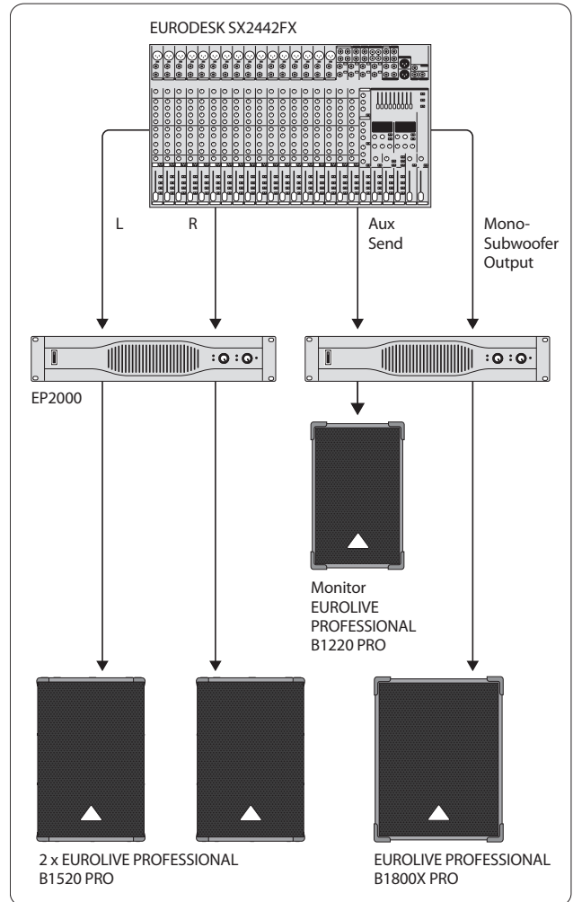
图 6.1: 带舞台监听音箱和超低音扬声器的立体声运行
