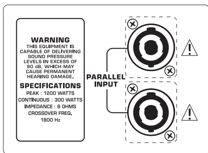
图 1.1: B1520 PRO 的连接区 (B1220 PRO/B2520 PRO 相似)
