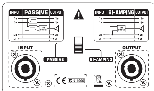
图 1.2: 超低音箱 (B1800X PRO) 的连接区
