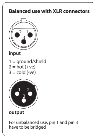
Рис. 4.3: Соединения XLR
