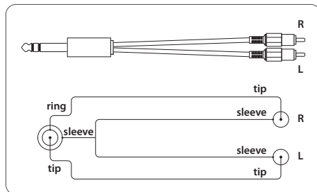
Рис. 4.4: Адаптерный кабель стерео
