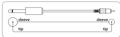
Рис. 4.5: Адаптерный кабель моно
