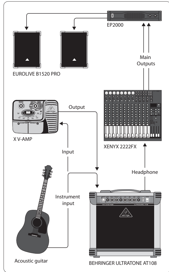
Рис. 2.2: Установка для „живых“ выступлений
