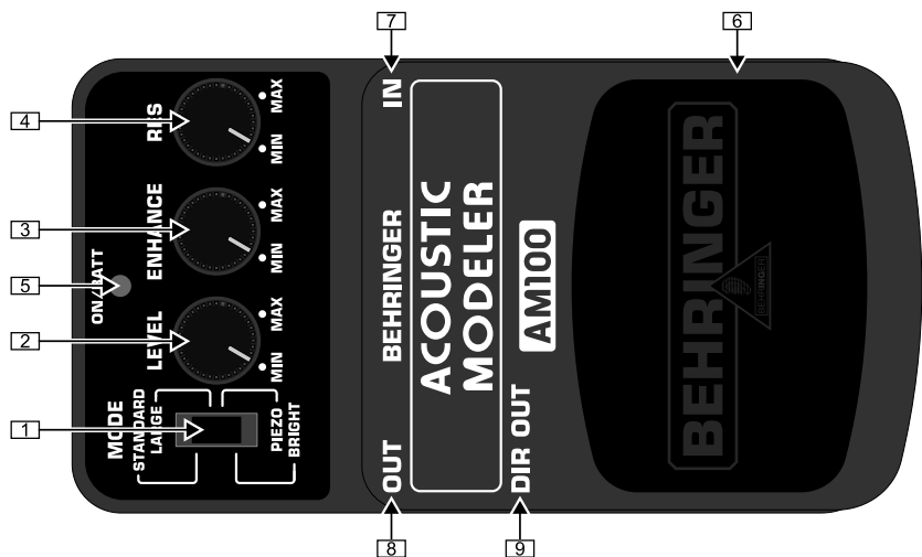
上面図
