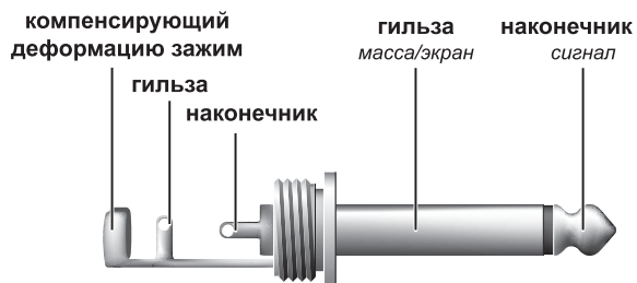
Рис. 5.3: 6,3 мм-монохраповый штекер
