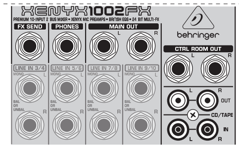
Afb. 2.3: De aansluitingen van de Main-sectie
