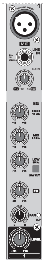
Afb. 2.1: De aansluitingen en regelaars van de monokanalen
