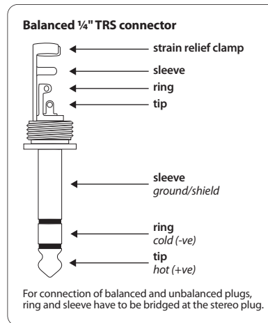
Afb. 4.3: 6,3-mm-stereoklinkerstekker
